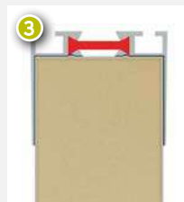
Profils haut à rupture de pont thermique
